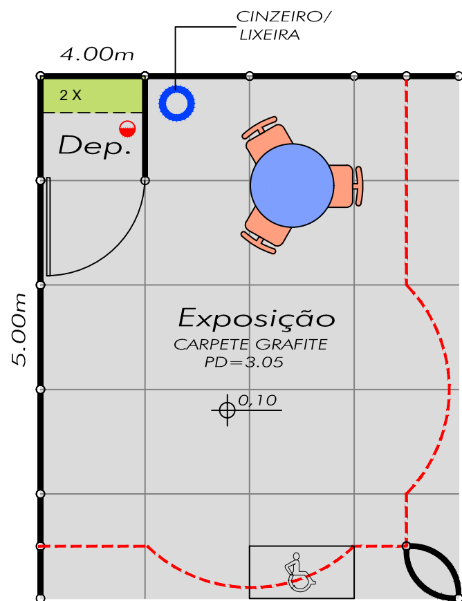
PLANTA ESC. 1/50
