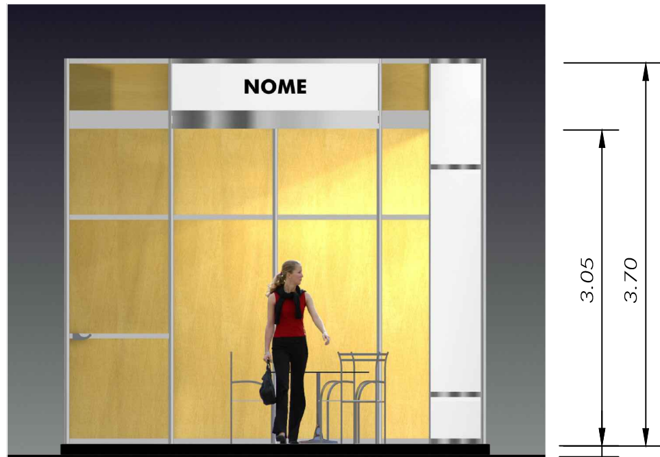
ELEVAÇÃO
