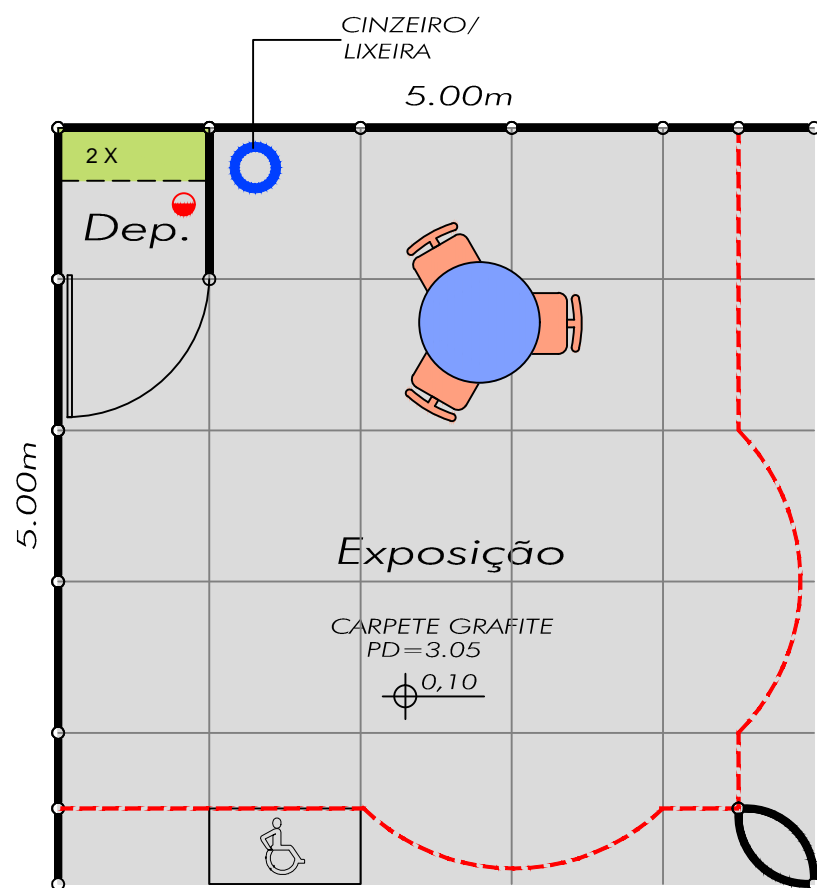
PLANTA ESC. 1/50
